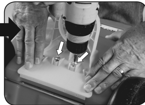
13 Person 1: Center and hold trailer hitch-bottom (I) securely on Cozy Coupe. Person 2: Install screws (L) x 2 in locations shown. Personne 1 : Centrez et tenez fermement le bas de l'attelage de la remorque (I) sur le Cozy Coupe. Personne 2 : Installez les deux vis (L) aux emplacements indiqués. Persona 1: Centre y sostenga bien el enganche inferior (I) en el Cozy Coupe. Persona 2: Instale 2 tornillos (L) en los lugares indicados.
