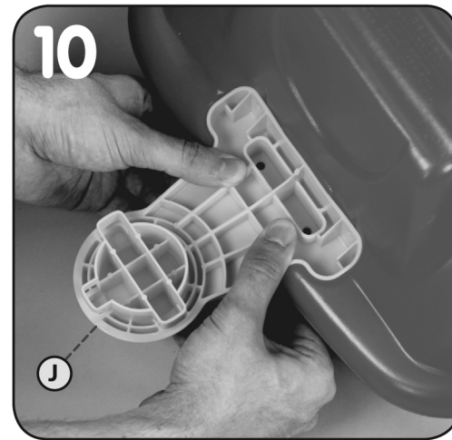
10 Snap trailer hitch-top (J) onto trailer as shown. Emboîtez le haut de l'attelage de la remorque (J) sur la remorque comme illustré. Encaje el enganche superior (J) en el remolque tal y como se muestra.
