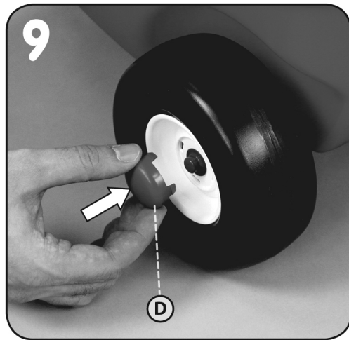
9 Align slots and snap on top hat covers (D) x 2. Alignez les fentes et emboîtez les capuchons de vis (D) x 2. Alinee las ranuras y encaje las 2 cubiertas de remates (D).
