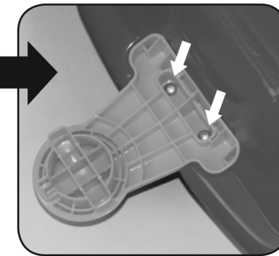
11 To secure, install screws (L) x 2 in locations shown. Pour fixer, installez les deux vis (L) aux emplacements indiqués. Para fijarlo instale 2 tornillos (L) en los lugares indicados
